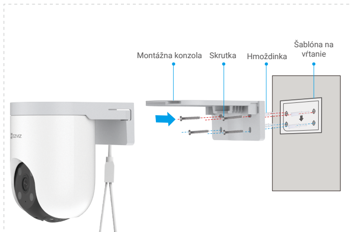
Obr. 2 Nástenné upevnenie
