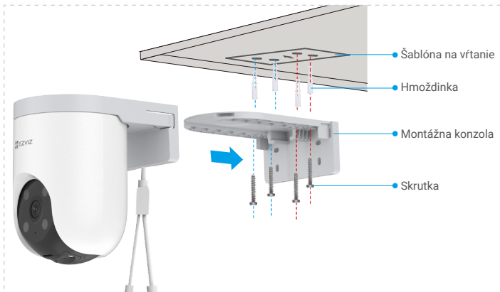
Obr. 1 Stropné upevnenie
